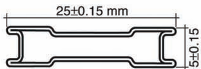
ANODIZADO BRONCE
